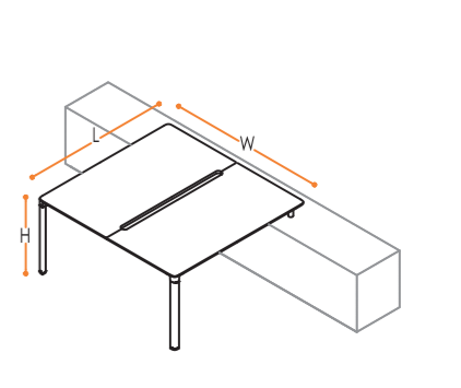
ETAJER VE KONSOLA BAĞLANAN GRUP MASALAR W:160 DOUBLE GROUP TABLES ASSEMBLED TO CONSOLLE / BENCH
