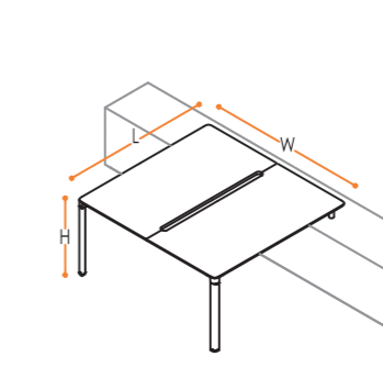
ETAJER VE KONSOLA BAĞLANAN GRUP MASALAR W:140 DOUBLE GROUP TABLES ASSEMBLED TO CONSOLLE / BENCH
